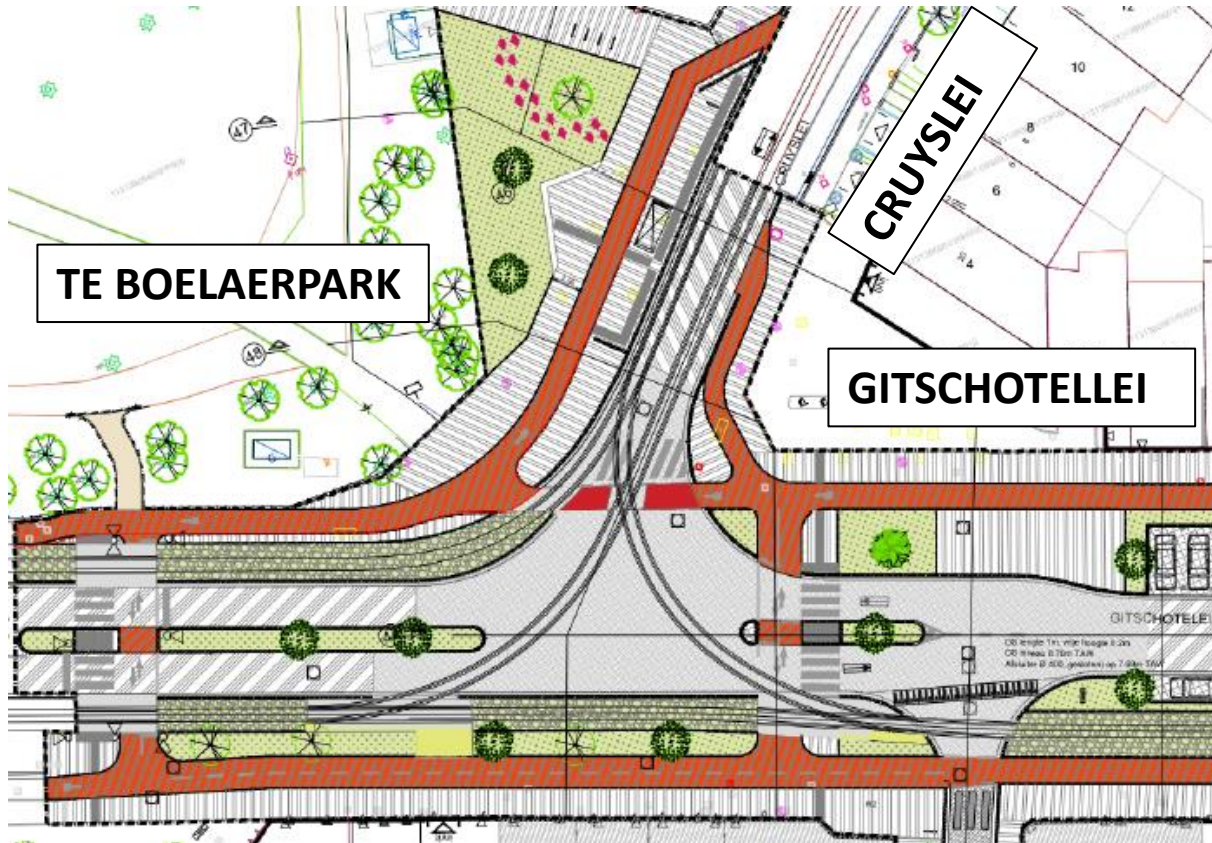
Kruispunt Gitschotellei-Cruyslei
