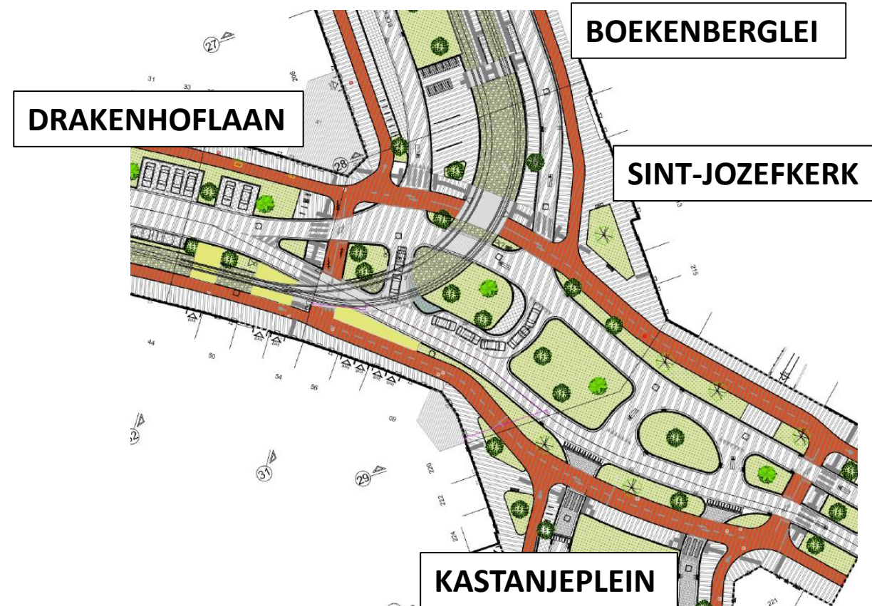
Kruispunt Drakenhoflaan-Boekenberglei
