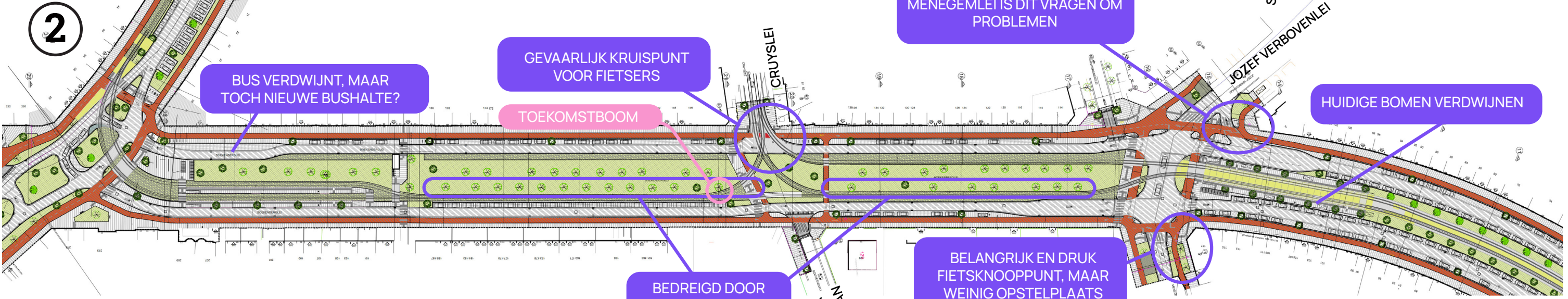
Grondplan nieuwe toestand: Gitschotellei-Drakenhoflaan
